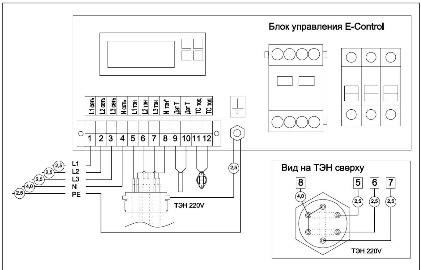
Рис. 4 - Подключение блока ТЭН (3 трубки по 220в) к трехфазной сети 380в.
