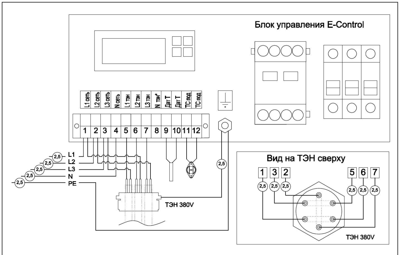
Рис. 3 - Подключение блока ТЭН (3трубки по 380в) к трехфазной сети 380в
