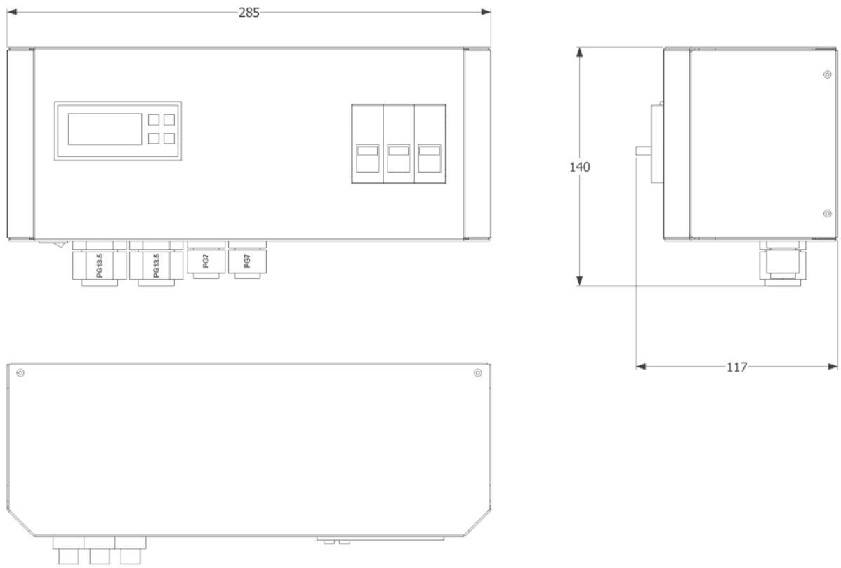
Рис. 1 - Габаритные размеры БУ
